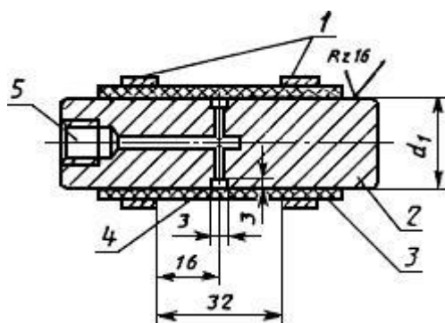
Черт.5. Установка шлангов наружным диаметром соответствующего хомута на проверочную оправку
